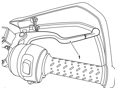
1. Palanca del freno delantero (se muestra Scrambler 400 X)
