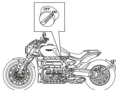
Hauptzündschalter
