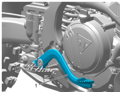
1. Hinterrad-Bremspedal
