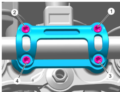
Anzugssequenz der Lenkerklemme (Position mit vergrößerter Reichweite)
